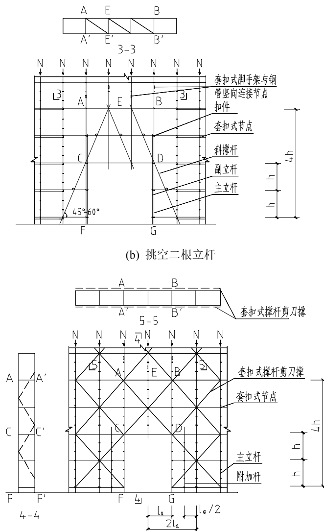
图 6.2.7 门洞处上升斜杆、平行弦杆桁架
