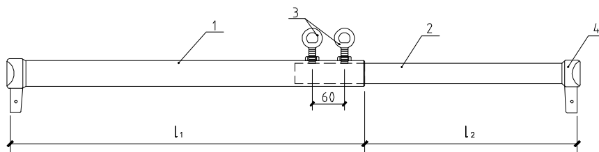
图 3.1.4 可调水平杆 1—外杆；2—内杆；3—紧固螺栓；4—水平杆端接头
