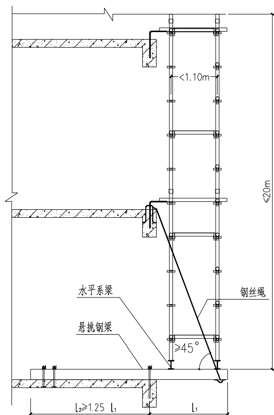
图 6.2.8-1 型钢悬挑脚手架构造
