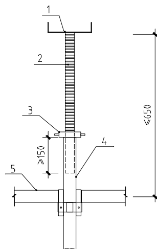
图 6.1.10-2 可调托座伸出顶层水平杆的长度
