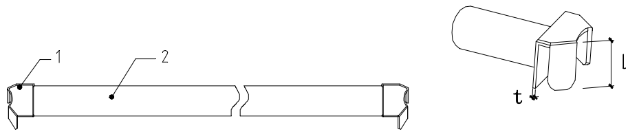
图 3.1.10 水平斜撑杆 1—专用端接头；2—钢管
