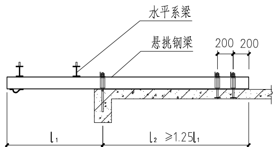
图 6.2.8-2 悬挑钢梁楼面构造
